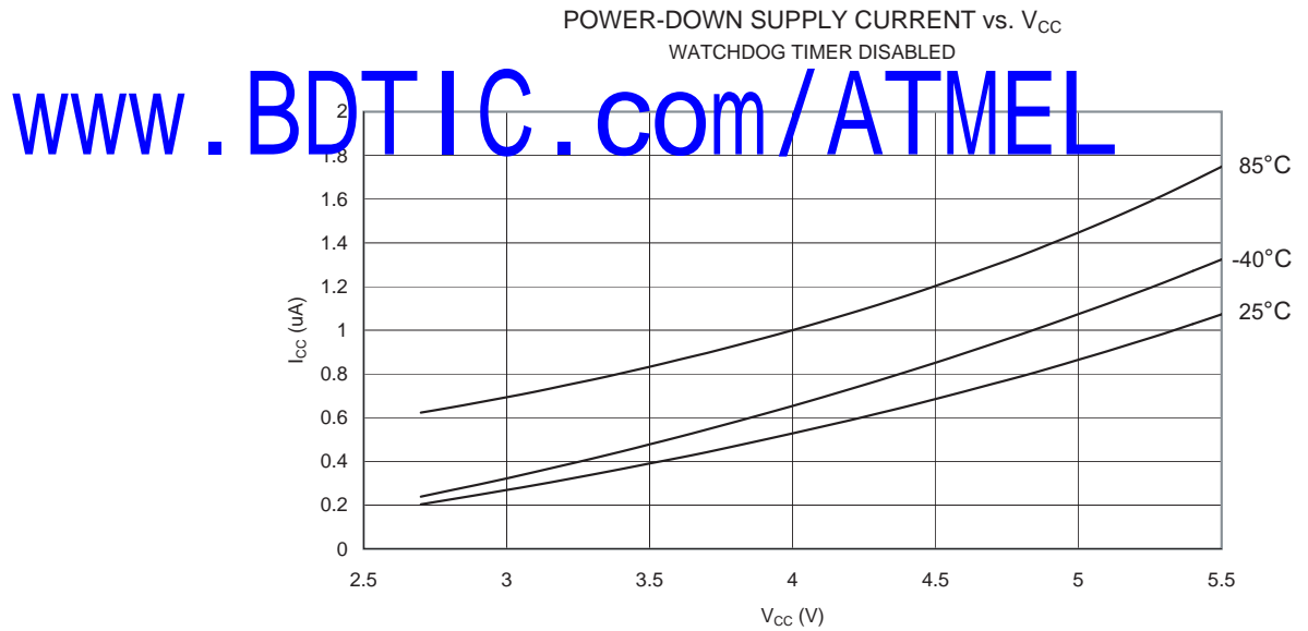
Figure 107. 掉电模式电流和 V_{CC} 的关系 (看门狗定时器禁用)
