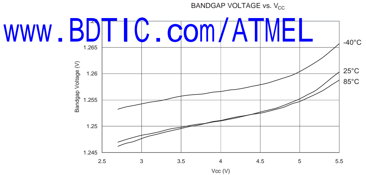
Figure 133. 能隙电压和 V_{CC} 的关系
