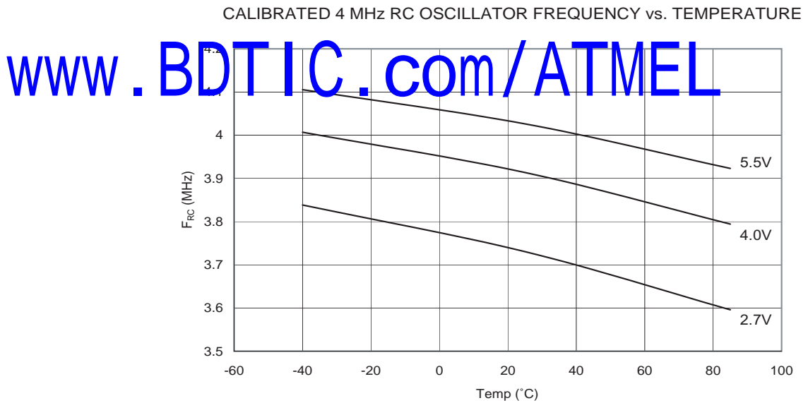
Figure 141. 校准的 4 MHz RC 振荡器频率和温度的关系
