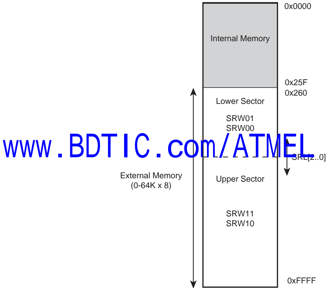
Figure 11. 可分区选择的外部存储器
