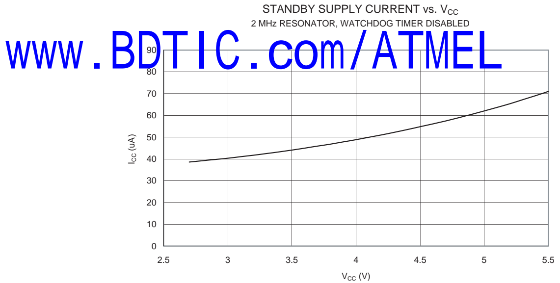
Figure 111. Standby 模式电流和 V_{CC} 的关系 (2 MHz 谐振器, 看门狗定时器禁用)
