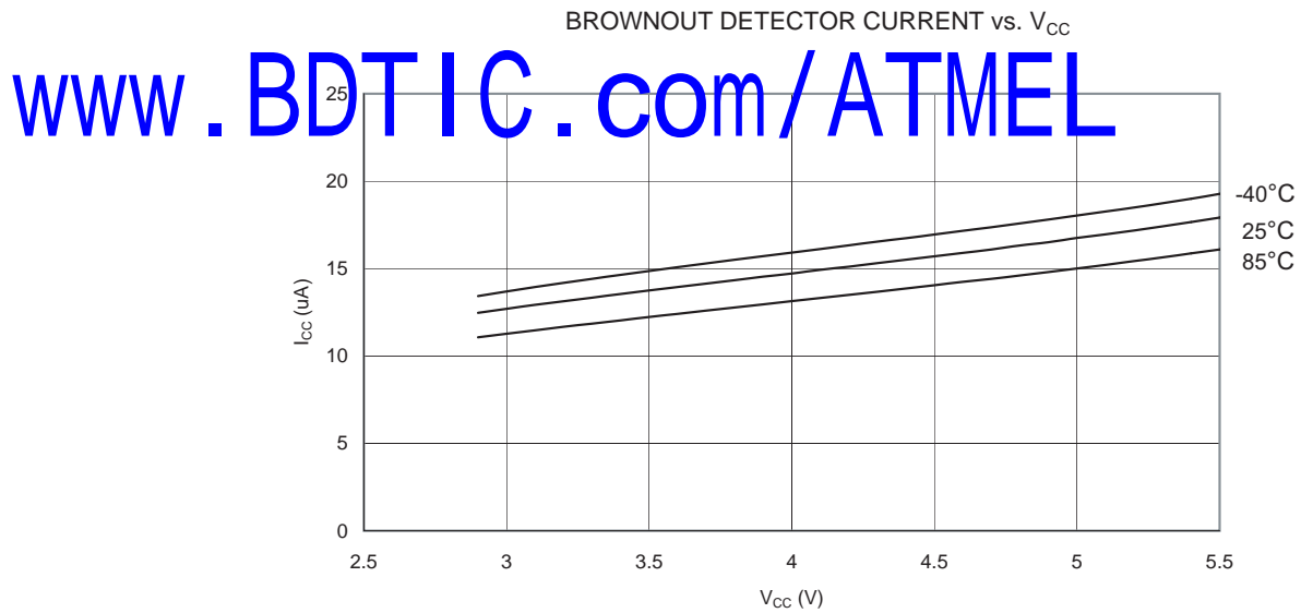
Figure 151. BOD 电流和 V_{CC} 的关系
