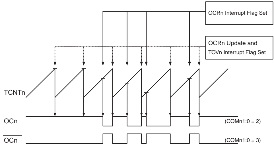
Figure 39. 快速 PWM 模式时序图
