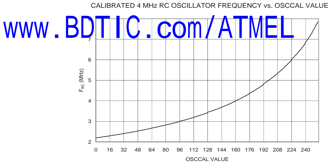
Figure 143. 校准的 4 MHz RC 振荡器频率和 Oscal 数值的关系
