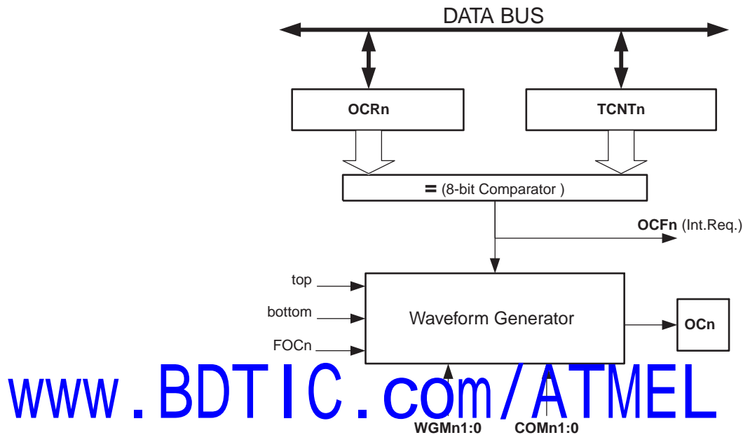
Figure 36. 输出比较单元方框图
