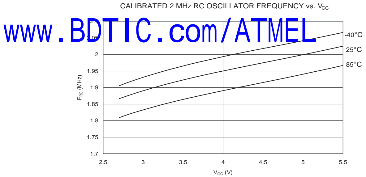
Figure 145. 校准的 2 MHz RC 振荡器频率和 V_{CC} 的关系
