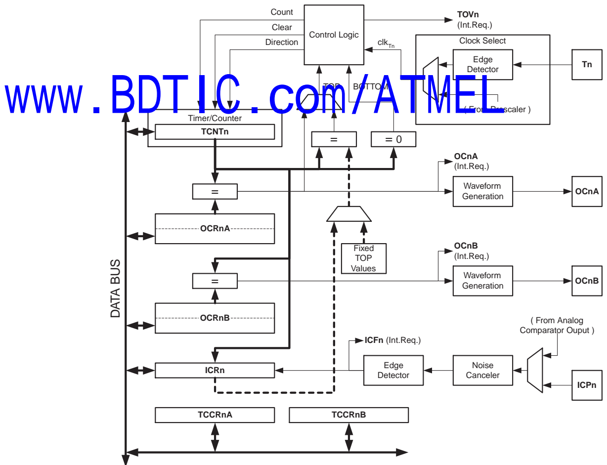
Figure 47. 16 位 T/C 框图 (1)
