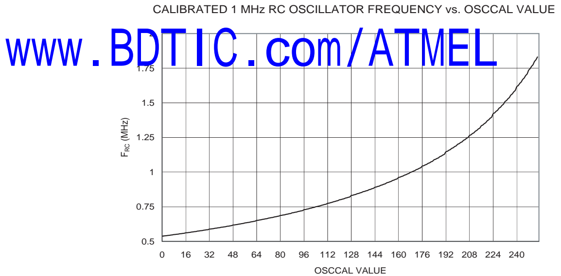
Figure 149. 校准的 1 MHz RC 振荡器频率和 Oscal 数值的关系
