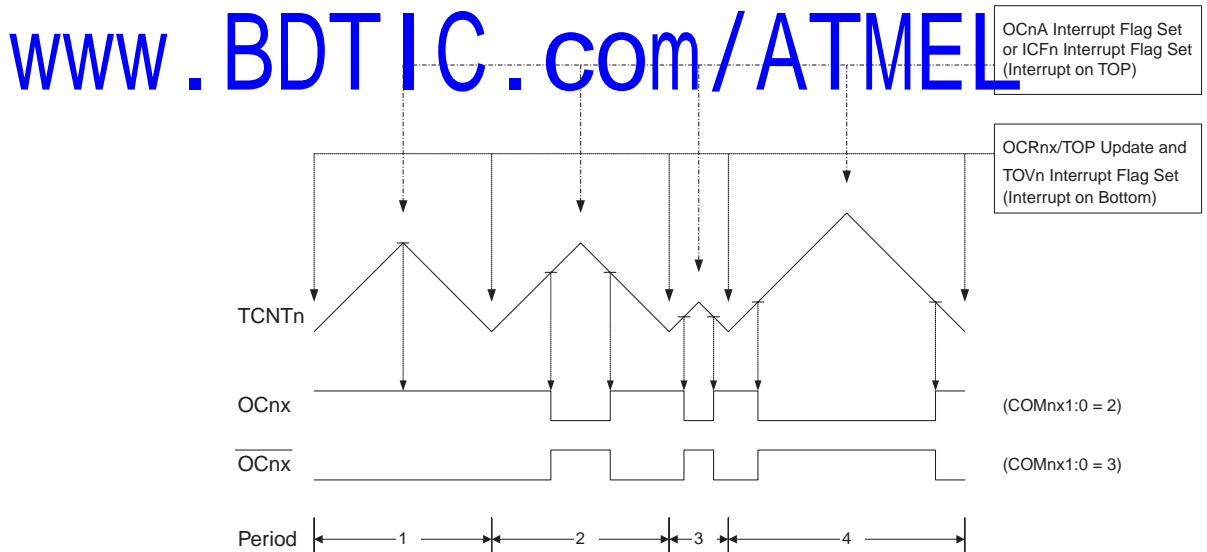
Figure 55. 相位与频率修正 PWM 模式的时序图
