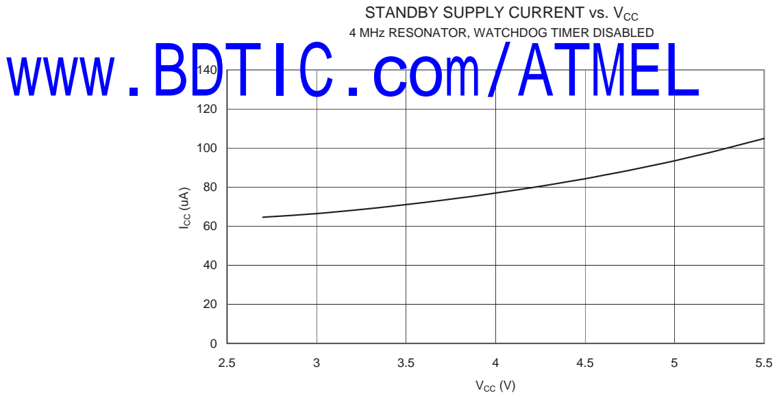
Figure 113. Standby 模式电流和 V_{CC} 的关系 (4 MHz 谐振器 , 看门狗定时器禁用 )
