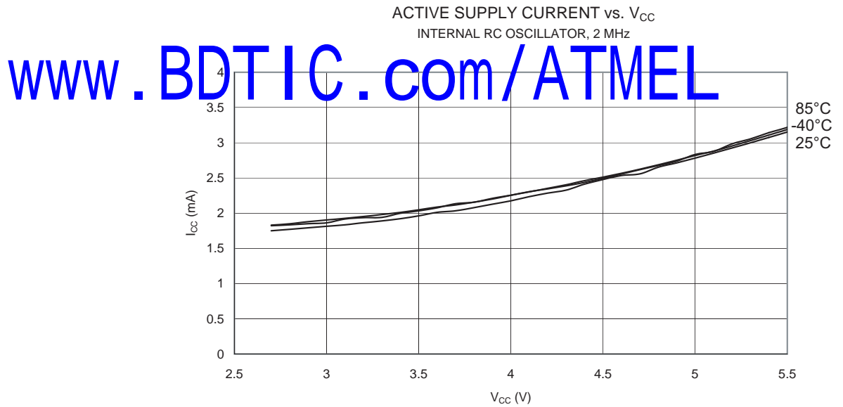
Figure 97. 工作电流和 V_{CC} 的关系 ( 内部 RC 振荡器 , 2 MHz)
