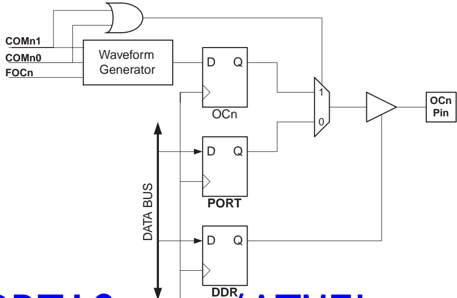
Figure 37. 比较匹配输出单元原理图
