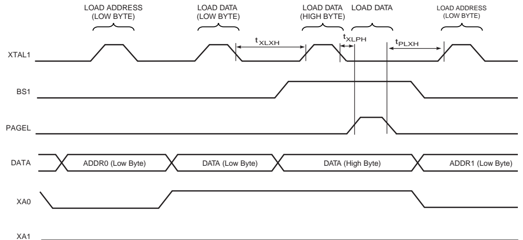
Figure 82. 并行编程时序，有时序要求的加载序列 (1)
