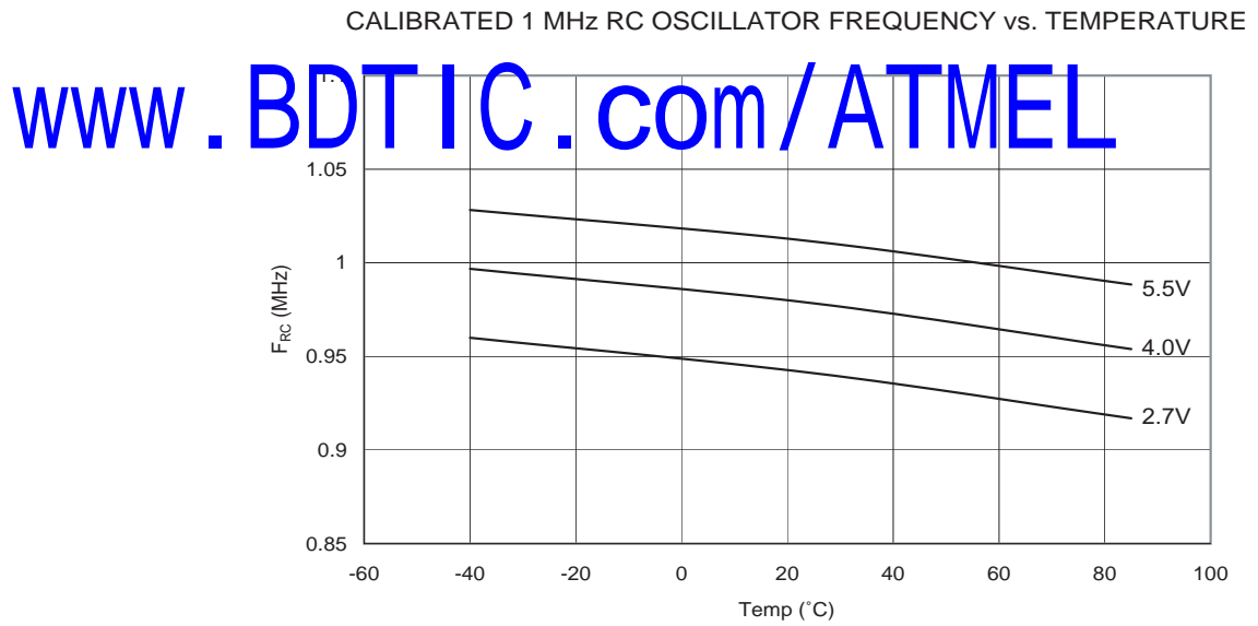
Figure 147. 校准的 1 MHz RC 振荡器频率和温度的关系
