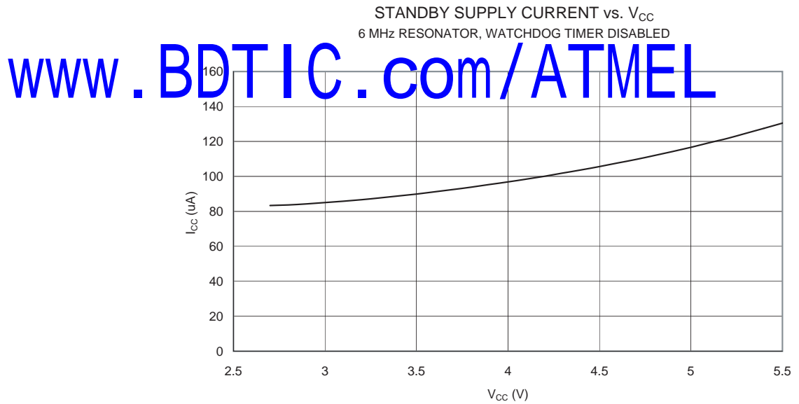
Figure 115. Standby 模式电流和 V_{CC} 的关系 (6 MHz 谐振器 , 看门狗定时器禁用)
