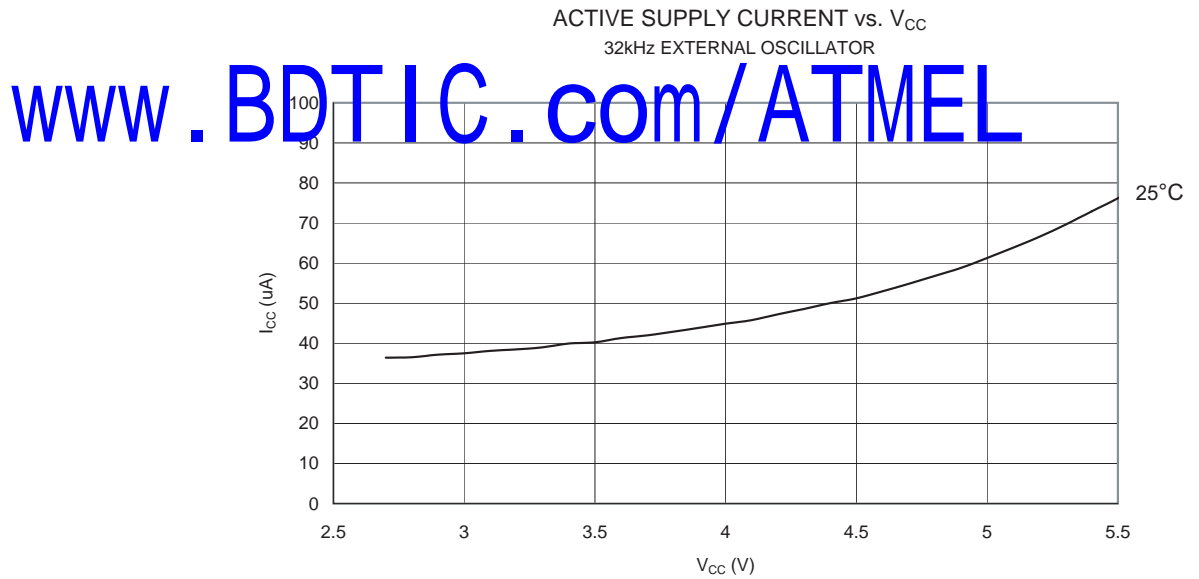
Figure 99. 工作电流和 V_{CC} 的关系 (32 kHz 外部晶振)
