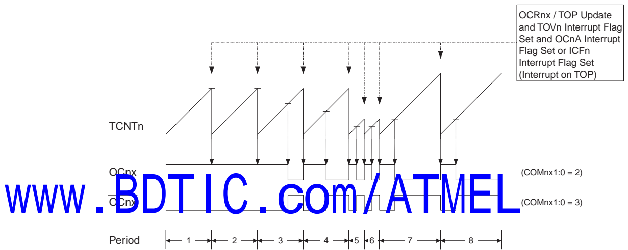
Figure 53. 快速 PWM 模式时序图
