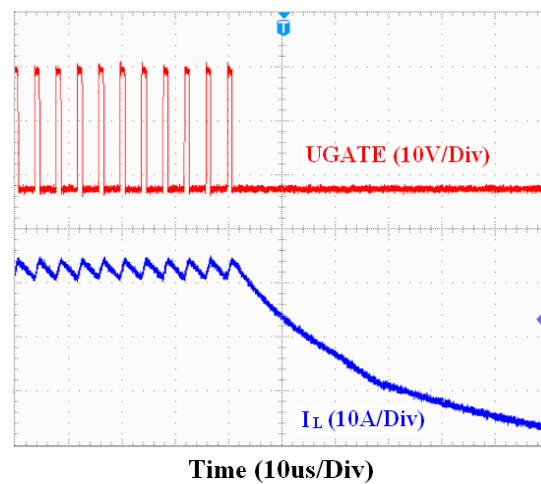
OCP
