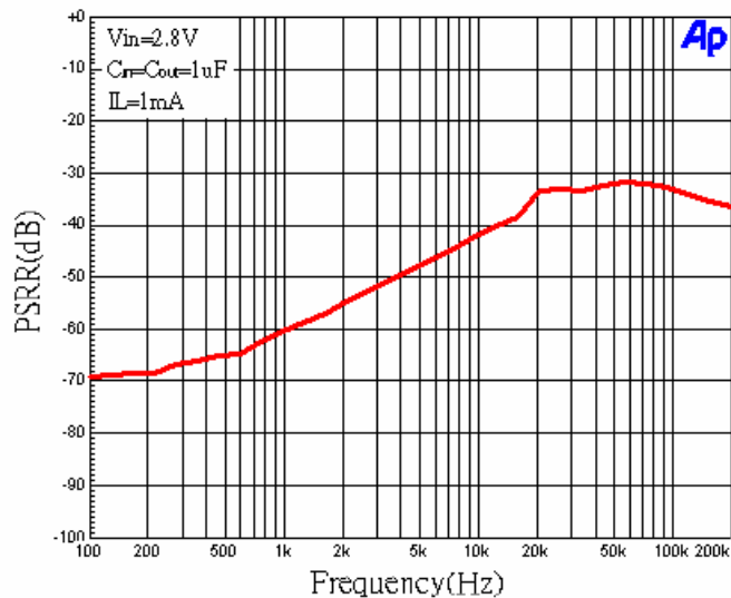
PSRR
