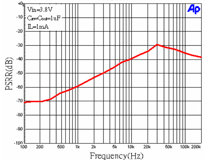
PSRR
