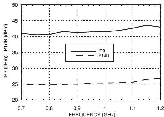
Output IP3 & P1dB
