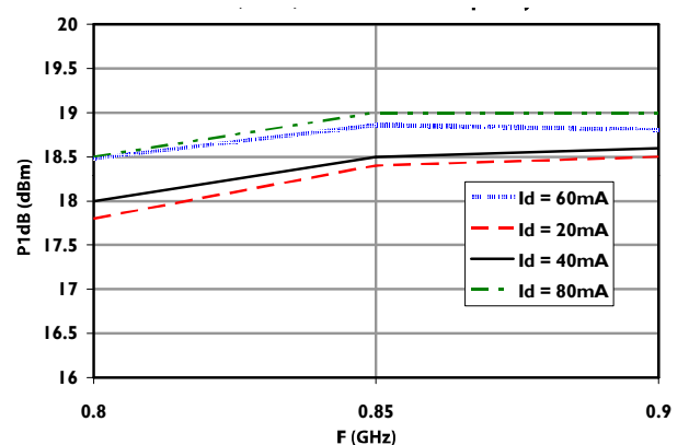
P1dB
