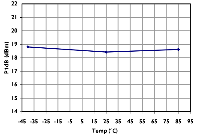
P1dB
