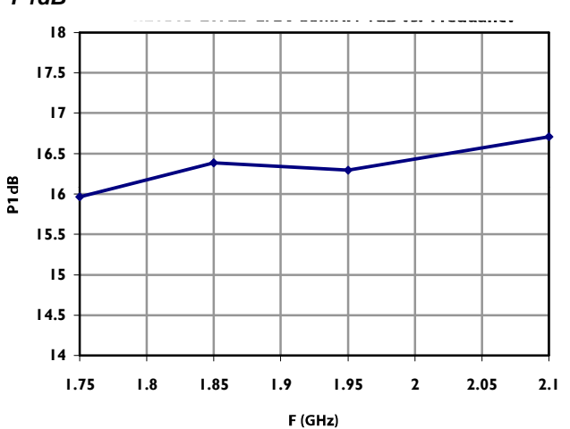
P1dB
