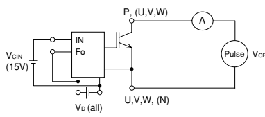
Fig. 4 I_{CES} Test
