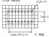
印刷基板加工尺寸 (TOP VIEW)
