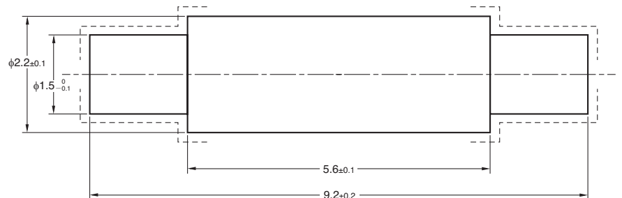
促动器设计参考图
