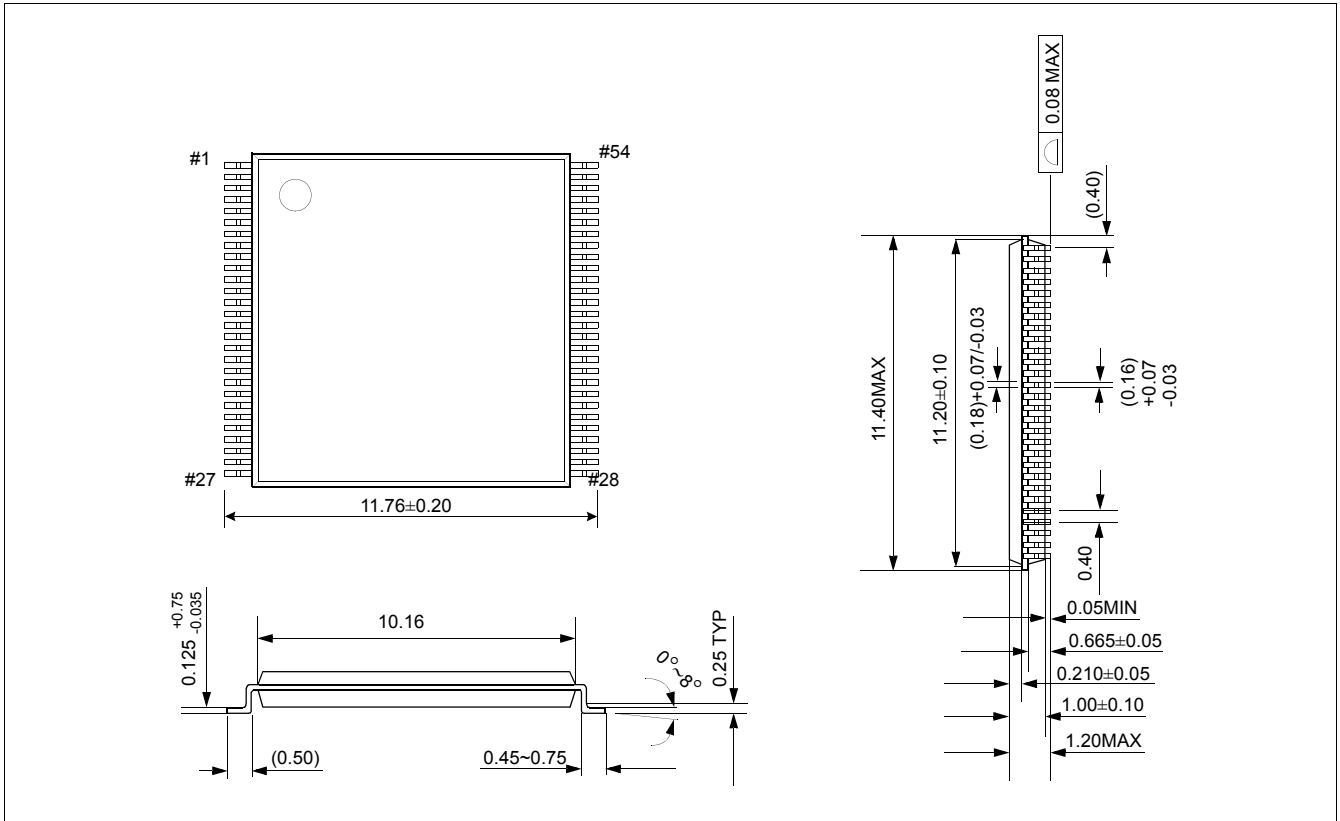
54pin sTSOPII-40 / Package dimension
