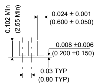
Detail Y
