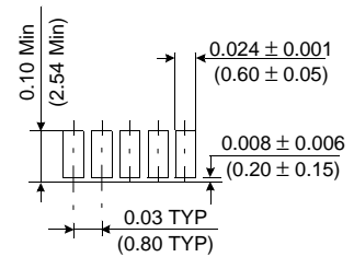
Detail Y
