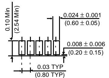
Detail Y
