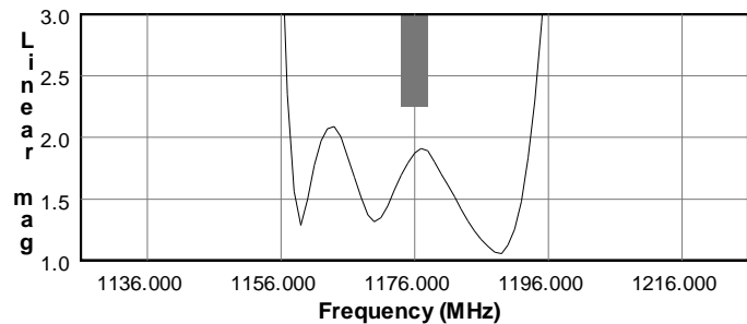
S11 VSWR
