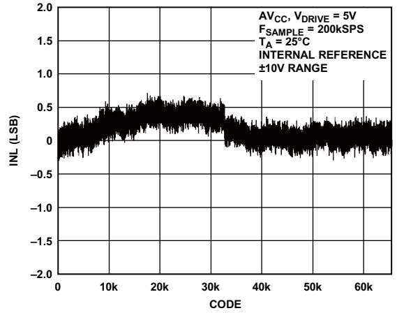
图14. AD7606典型INL, ±10 V范围
