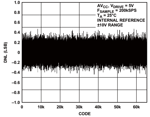
图15. AD7606典型DNL, ±10 V范围
