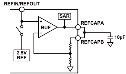
图40. 基准电压电路
