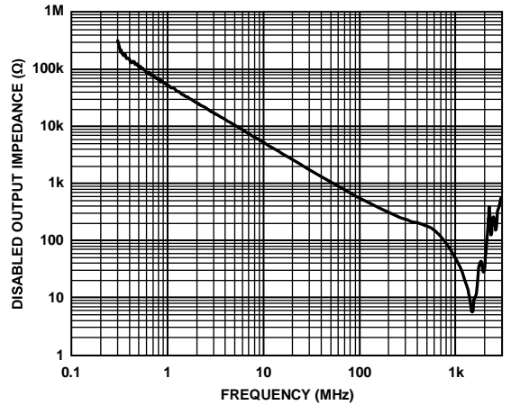
图46. ADV3222禁用输出阻抗
