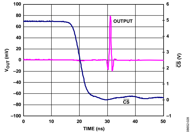
图22. ADV3222使能毛刺
