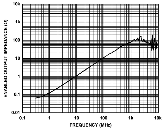
图47. ADV3222使能输出阻抗
