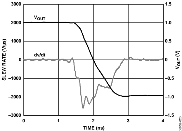
图14. ADV3221大信号下降压摆率 (3 pF负载、2 V峰峰值)
