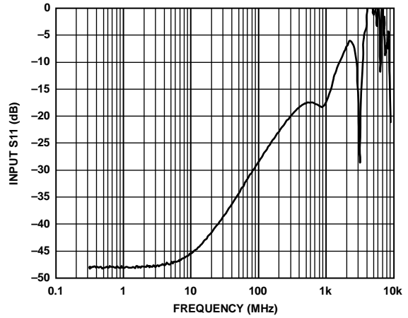
图45. ADV3221/ADV3222 S11 (包括评估板)
