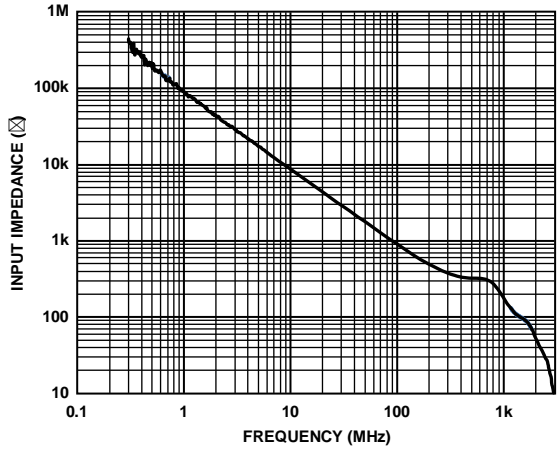
图42. ADV3221/ADV3222输入阻抗
