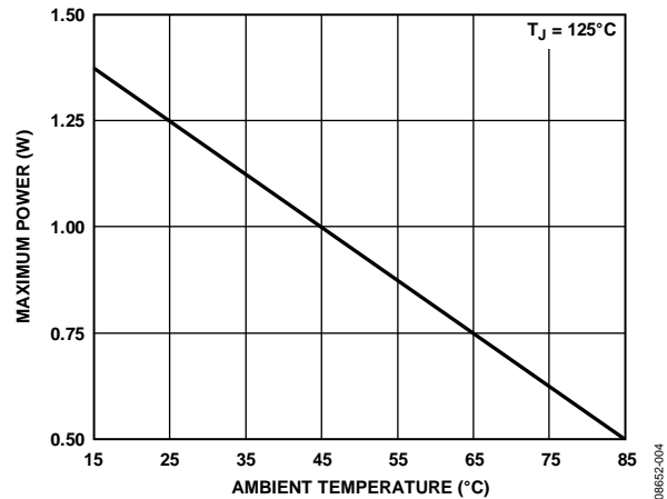
图4. 芯片最大功耗与环境温度的关系
