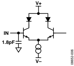
图54. ADV3221/ADV3222模拟输入
