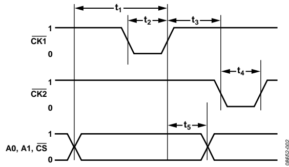
图2. 时序图
