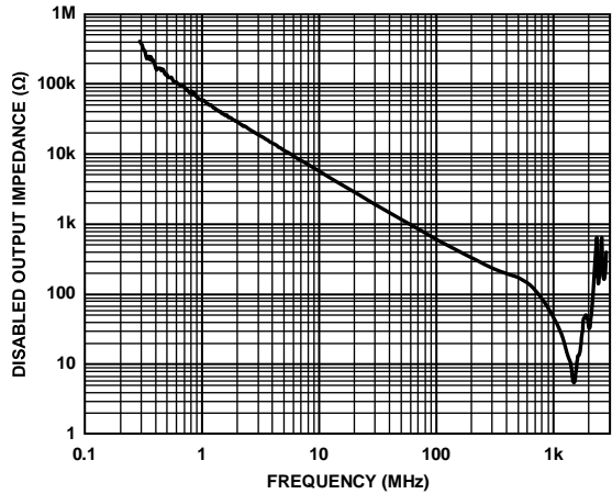
图43. ADV3221禁用输出阻抗
