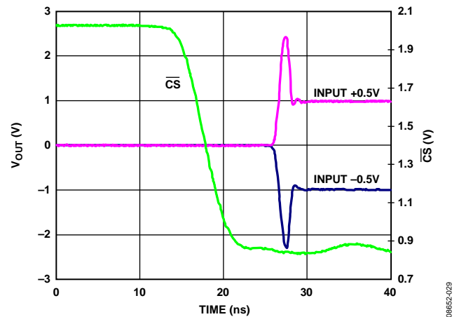
图23. ADV3222使能导通时序
