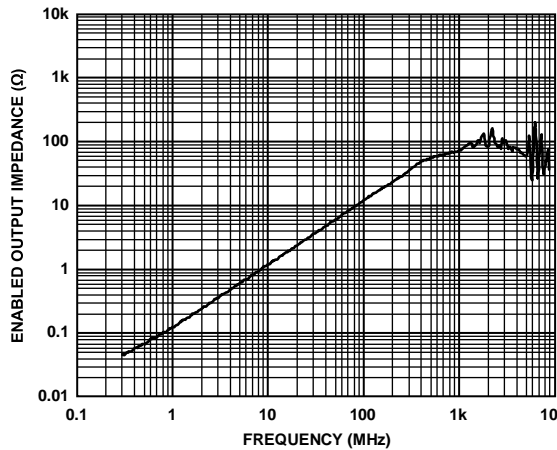
图44. ADV3221使能输出阻抗
