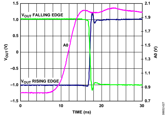
图21. ADV3222开关时间
