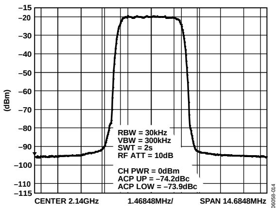
图15. 单WCDMA载波的频谱，中心频率 = 2140 MHz，载波功率 = 0 dBm，ACPR = -74 dBc
