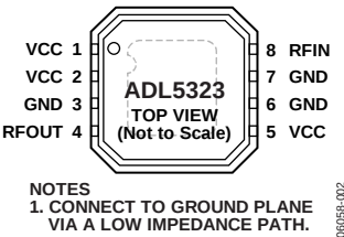
图3. 引脚配置
