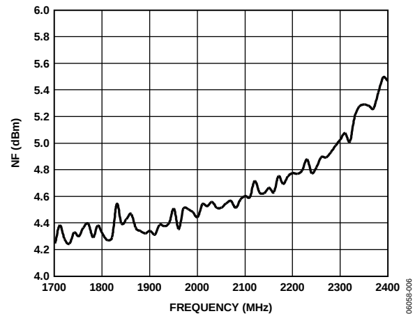
图7. 噪声系数与频率的关系, V_{CC} = 5\text{ V} , T_A = 25^\circ\text{C}
