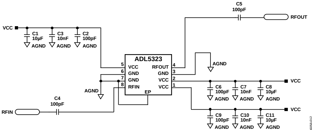
图17. 基本连接
