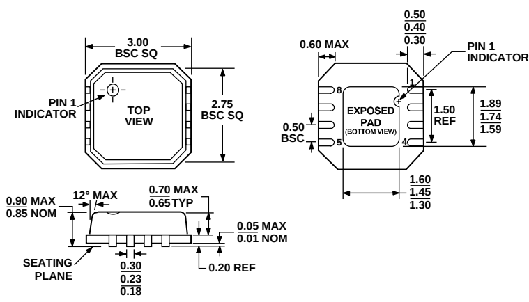
图20. 8引脚LFCSP_VD封装[引脚架构芯片级] 3 mm x 3 mm, 超薄体, 双列引脚 (CP-8-2) 尺寸单位: mm
