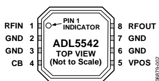
图2. 引脚配置
