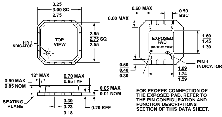
图21. 8引脚引线框芯片级封装[LFCSP_VD] 3 mm × 3 mm超薄体, 双列引脚 (CP-8-2) 图示尺寸单位: mm
