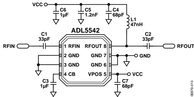
图14. 基本连接
