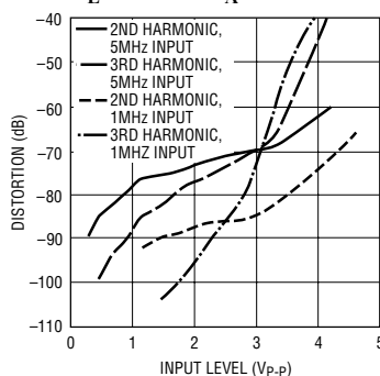
失真与信号电平的关系曲线 V_S = \pm 5V , 每个输出端上的 R_L = 800\Omega , T_A = 25^\circ C
