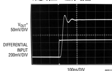
瞬态响应, 差分增益 = 1
