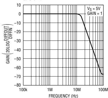
幅度响应
