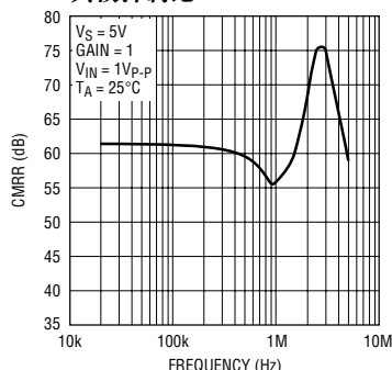
共模抑制比
