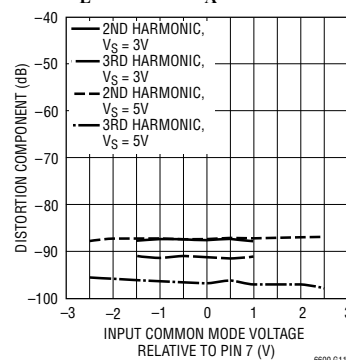
失真与输入共模电平的关系 曲线, 2V_{P-P} , 1MHz 输入, 1 倍增益, 每个输出端上的 R_L = 800\Omega , T_A = 25^\circ C
