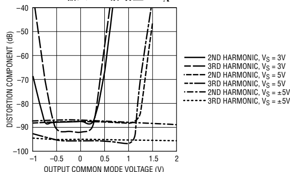
失真与输出共模电压的关系, 2V_{P-P} 1MHz 输入, 1 倍增益, T_A = 25^\circ C
