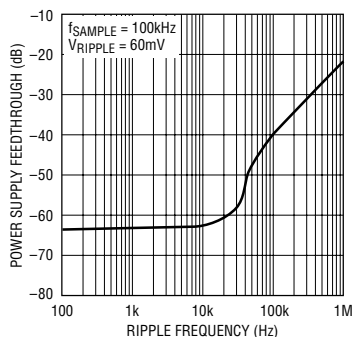
LTC1859 电源馈通与 纹波频率的关系曲线
