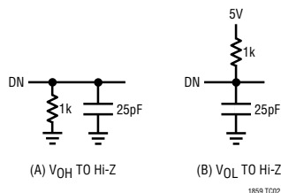
用于输出浮动延迟的负载电路
