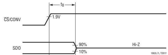
t 8 (BUS Relinquish Time)
