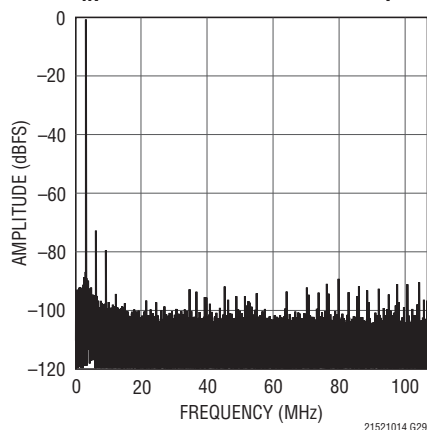
LTC2151-14: 32K Point FFT, f_{IN} = 417\text{MHz} , -1\text{dBFS} , 210Mps
