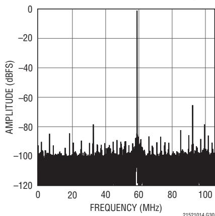
LTC2151-14: 32K Point FFT, f_{IN} = 571\text{MHz} , -1\text{dBFS} , 210Mps
