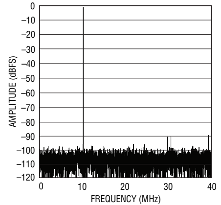
LTC2173-12: 8k Point FFT, f_{IN} = 70\text{MHz} -1\text{dBFS} , 80\text{Msps}
