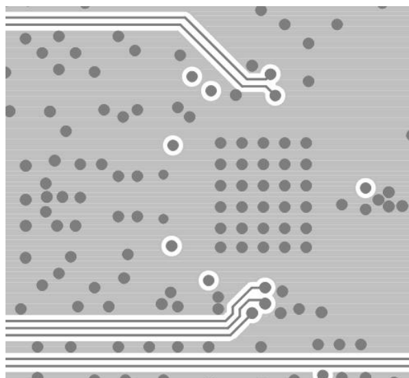
Inner Layer 3
