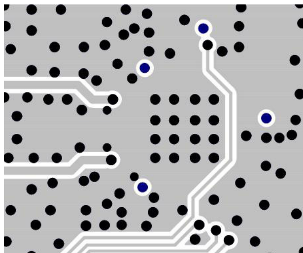
Inner Layer 4
