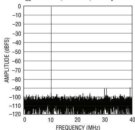
LTC2266-12: 8k Point FFT, f_{IN} = 70\text{MHz} , -1\text{dBFS} , 80\text{Mpsps}
