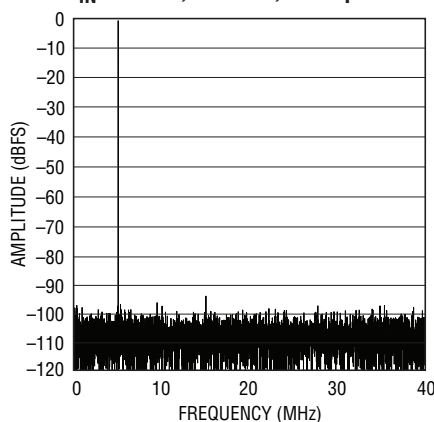
LTC2266-12: 8k Point FFT, f_{IN} = 5\text{MHz} , -1\text{dBFS} , 80\text{Mpsps}
