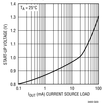
最小起动电压与负载电流的关系曲线
