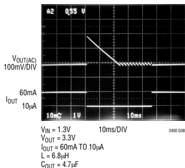
固定频率和突发模式操作
