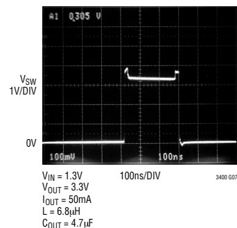
SW引脚固定频率、连续电感 器电流操作
