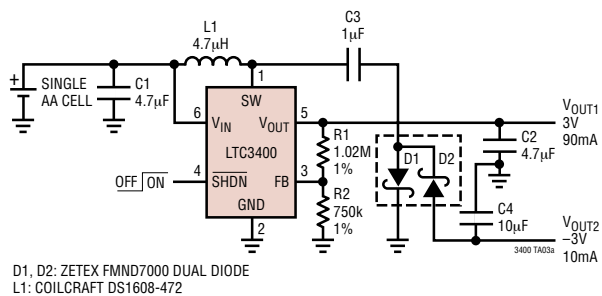
单节 AA 电池至 \pm 3V 同步升压型转换器
