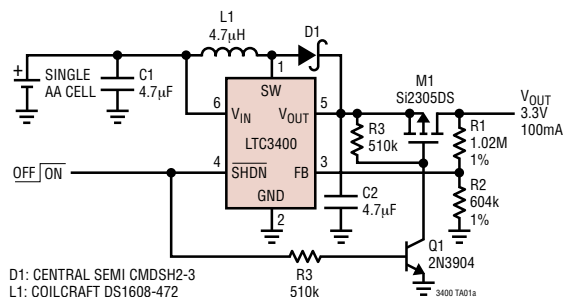
在停机状态下将负载断接的单节电池至 3.3V 同步升压型转换器
