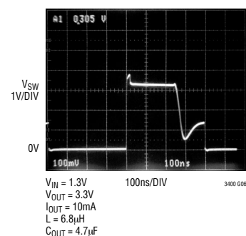
SW引脚抗振铃操作
