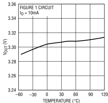
V_{OUT} 与温度的关系曲线
