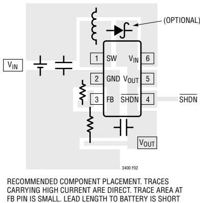
图 2：对单层电路板的推荐元件布置方案
