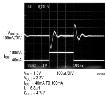
V_{OUT} 瞬态响应
