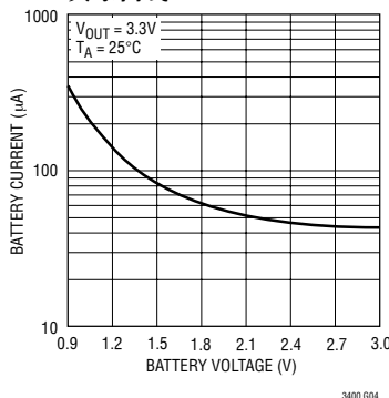
无负载电池电流与 V_{BATT} 的关系曲线
