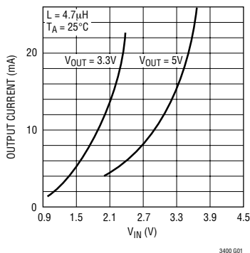
输出负载突发模式门限与 V_{IN} 的关系曲线
