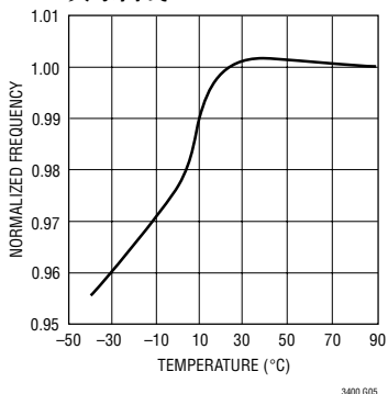
归一化振荡器频率与温度的关系曲线
