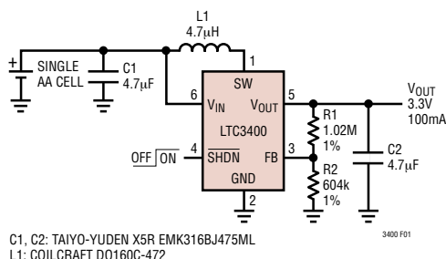
图1：单节电池至 3.3V 同步升压型转换器
