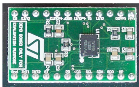
STEVAL-MKI084V1
