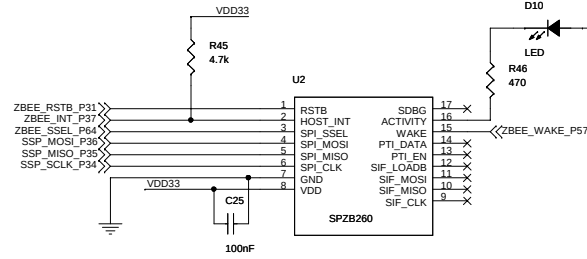
Zigbee Module
