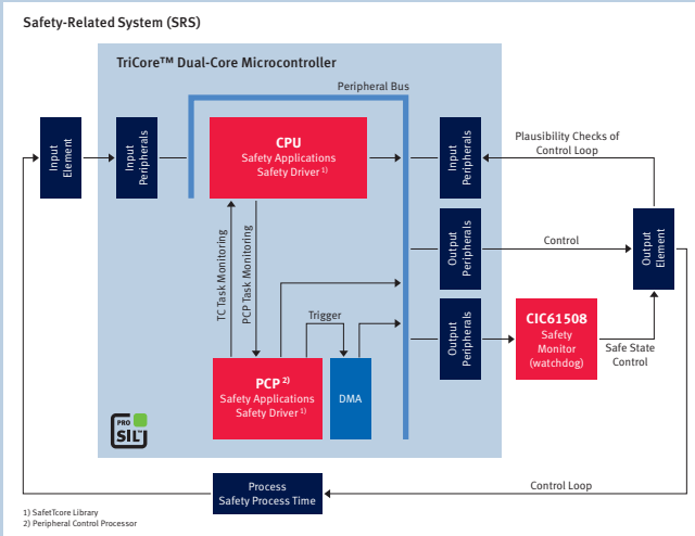
安全相关系统(SRS)结构框图
